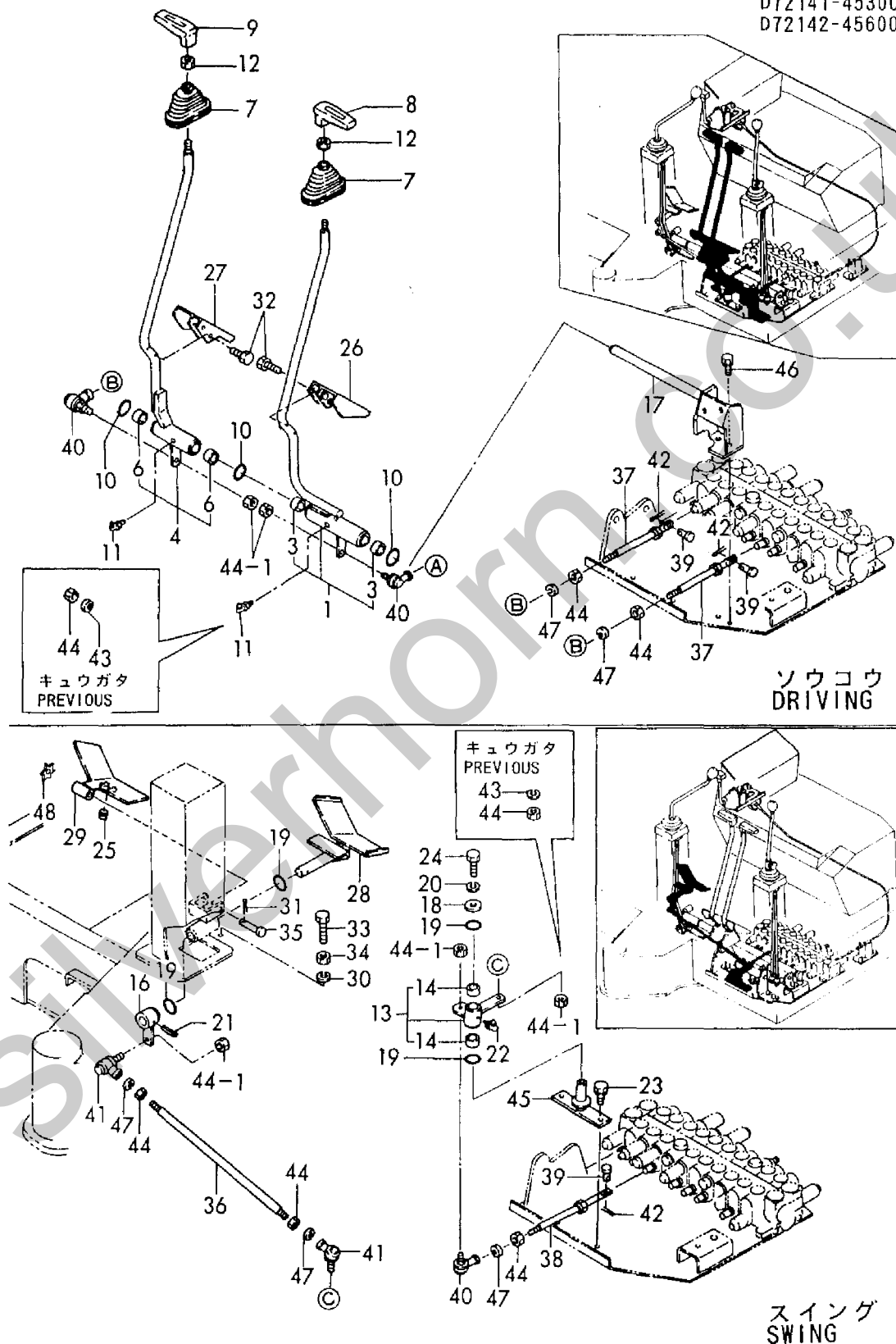
Fig. 27 ソウジュウソウチ(ソコウ & スイング) CONTROL EQUIP. (DRIVING & SWING)
