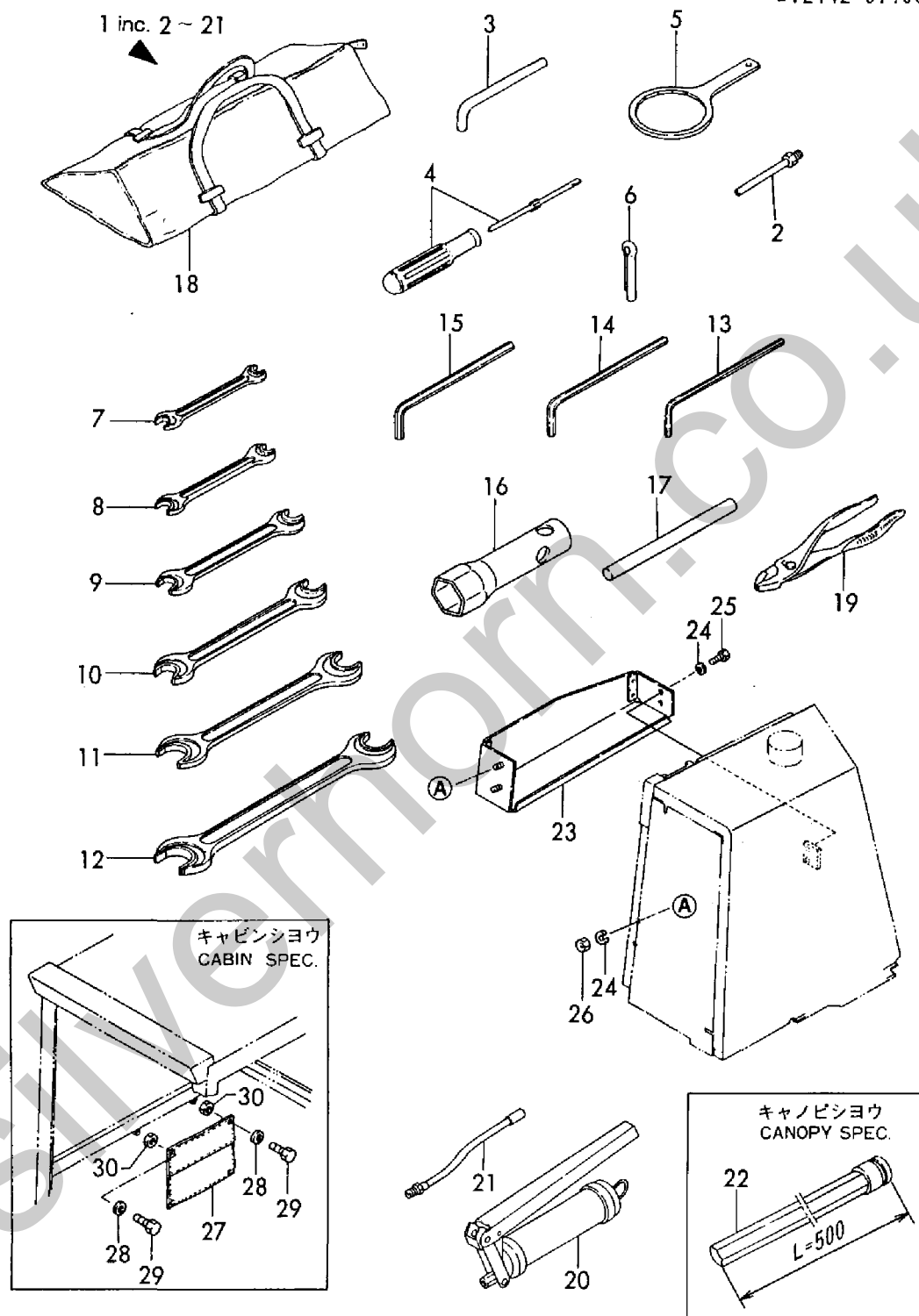
Fig. 5 コウグ, コウグバコ & マニュアルケース TOOL, TOOL BOX & MANUAL CASE
