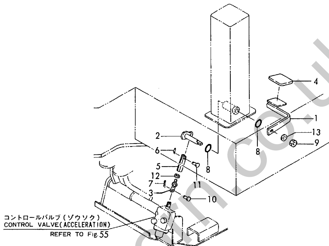
Fig. 21 ソウジュウソウチ (ゾウソクペダル) CONTROL EQUIP. (ACCELERATOR PEDAL) SPEC. CODE D72148-41700
