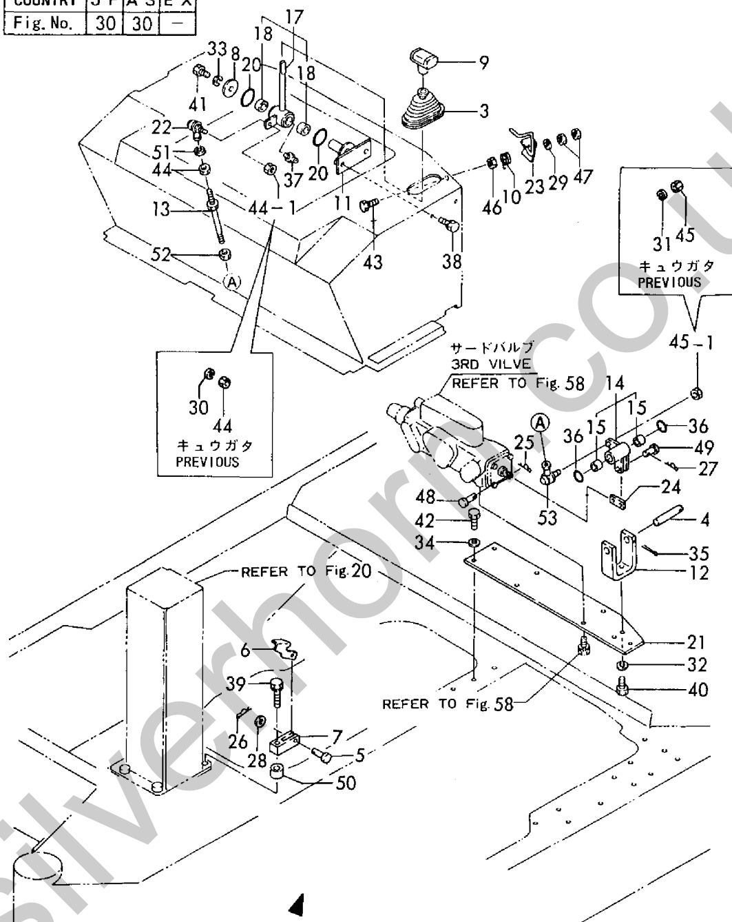
Fig. 30 ソウジュウソウチ (3RDバルブ) CONTROL EQUIP. (3RD VALVE)
