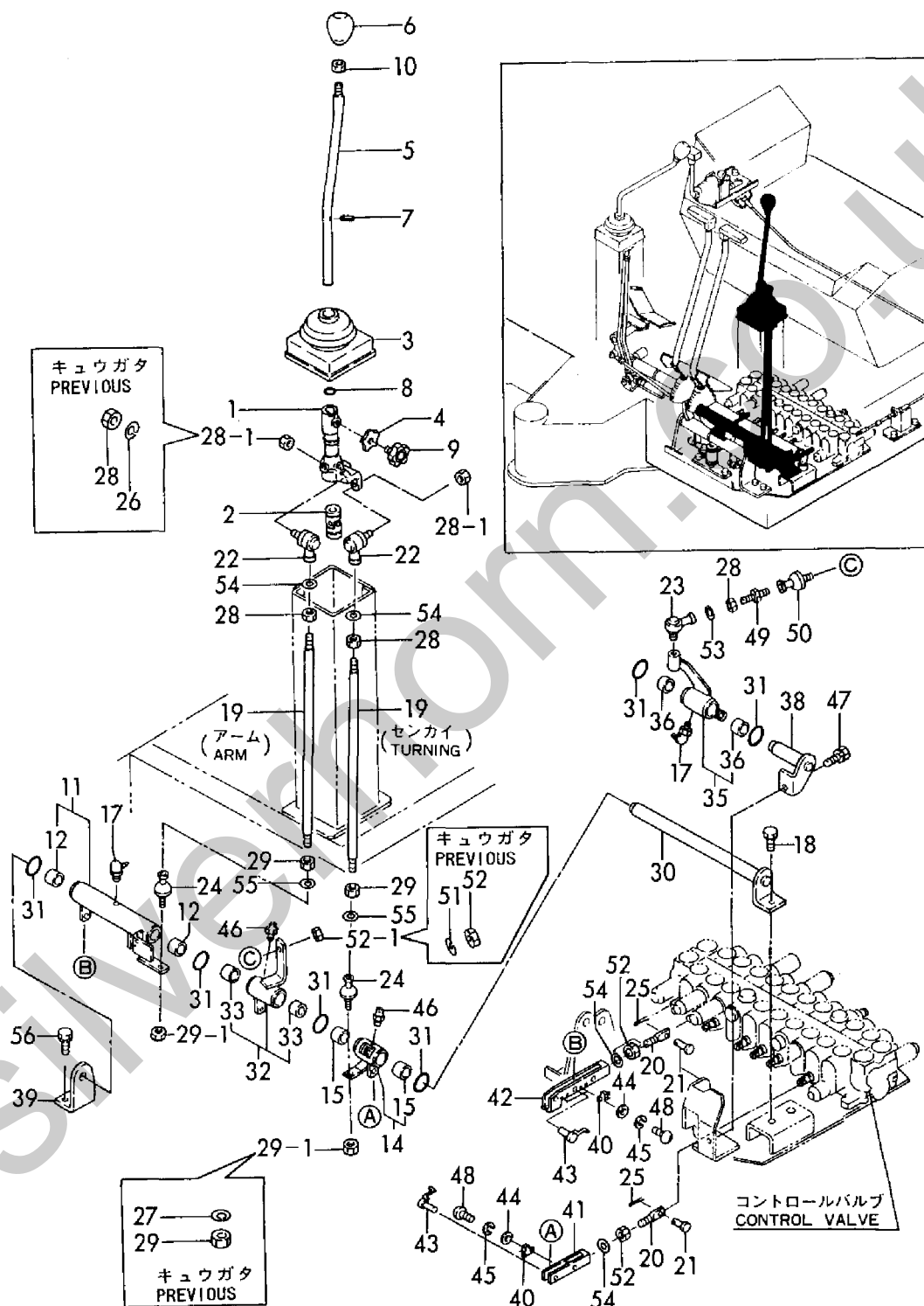
Fig. 26 ソウジュウソウチ(アーム & センカイ)(マルチタイプ) CONTROL EQUIP. (ARM & TURNING) (MULTI TYPE)
