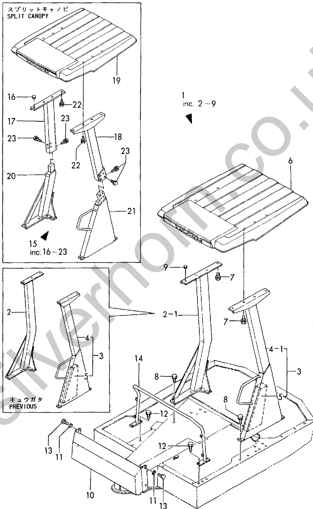
Fig. 38 キャノピ CANOPY
