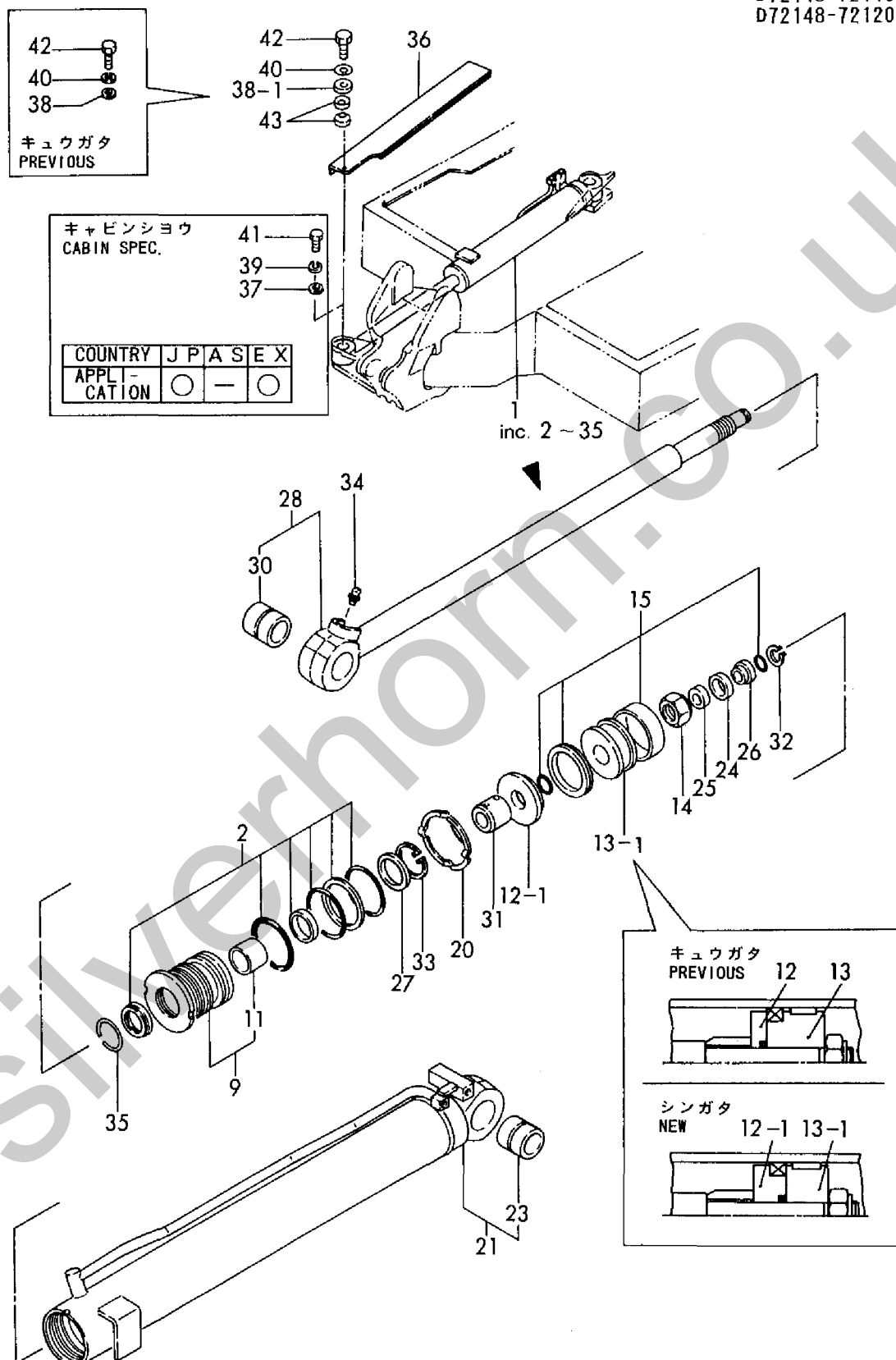
Fig. 45 スイングシリンダ SWING CYLINDER
