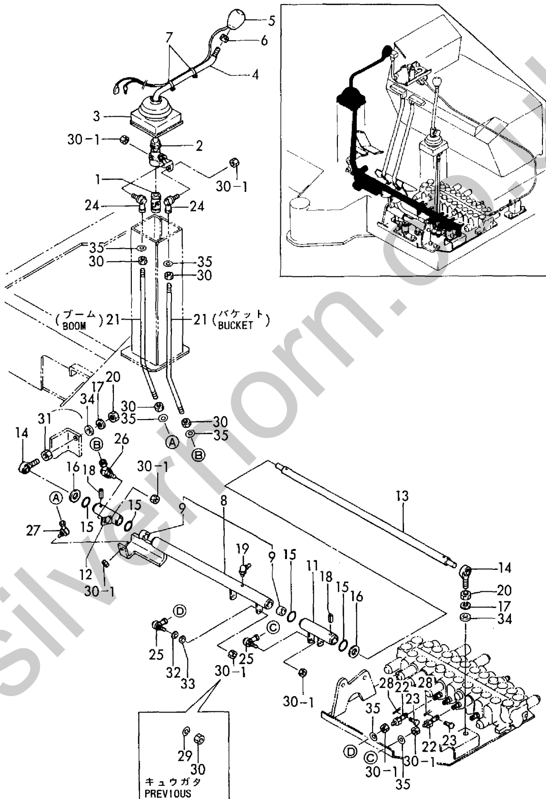
Fig. 22 ソウジュウソウチ(ブーム & バケット) CONTROL EQUIP. (BOOM & BUCKET)
