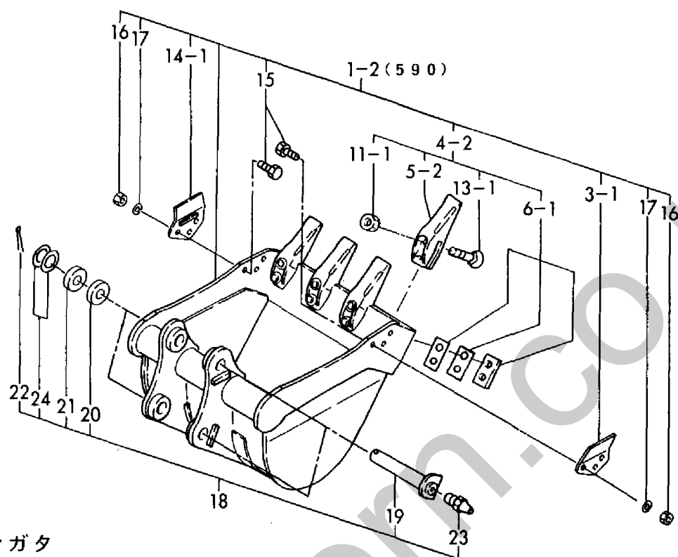
Fig. 71 バケット(550, 590) BUCKET(550, 590)
