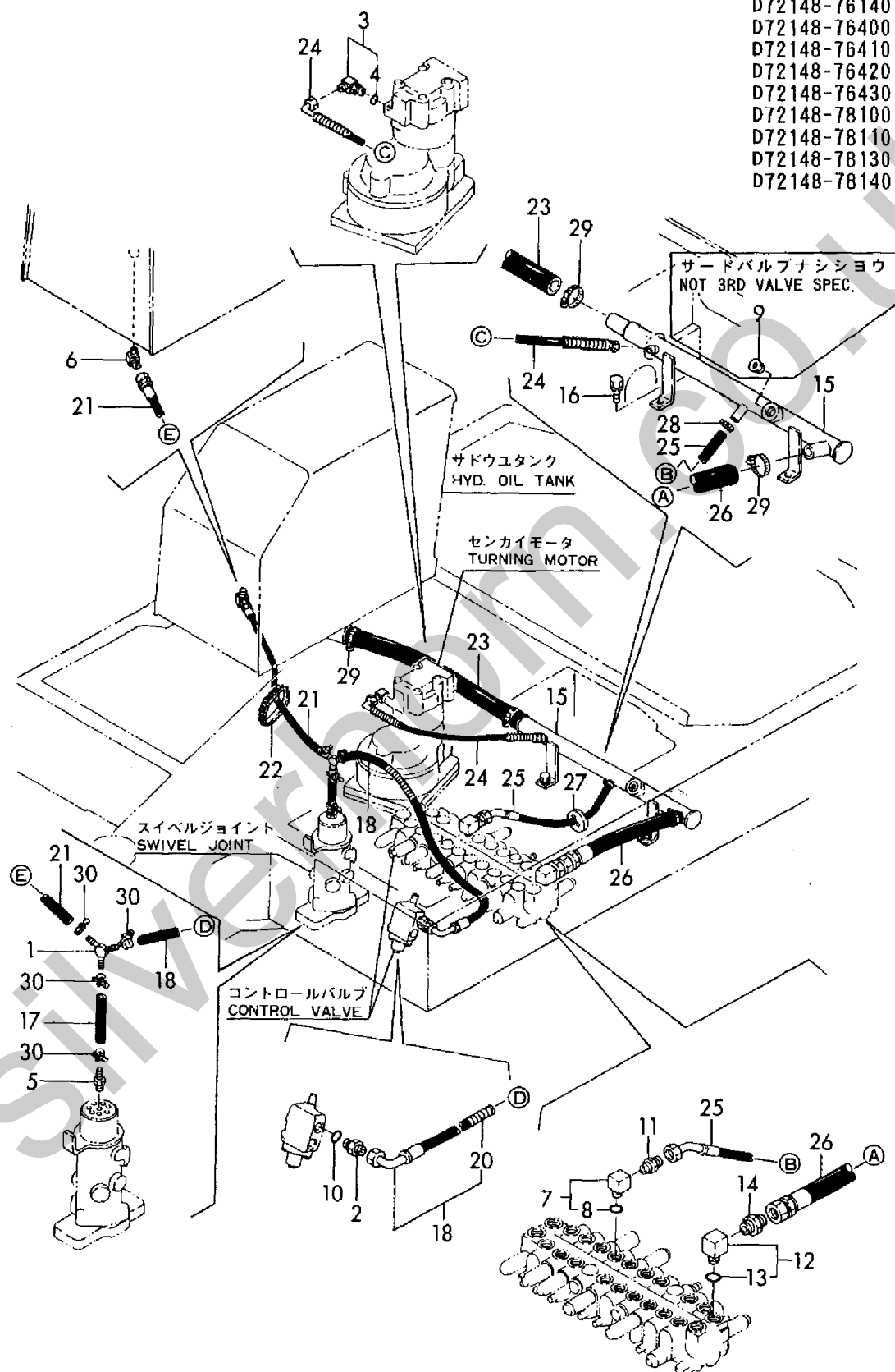
Fig. 64 ユアツハイカン(リターン) HYD. OIL PIPING(RETURN)
