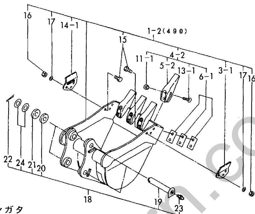
Fig. 73 バケット(450, 490)(7タッチメント) BUCKET(450, 490)(ATTACHMENT)
