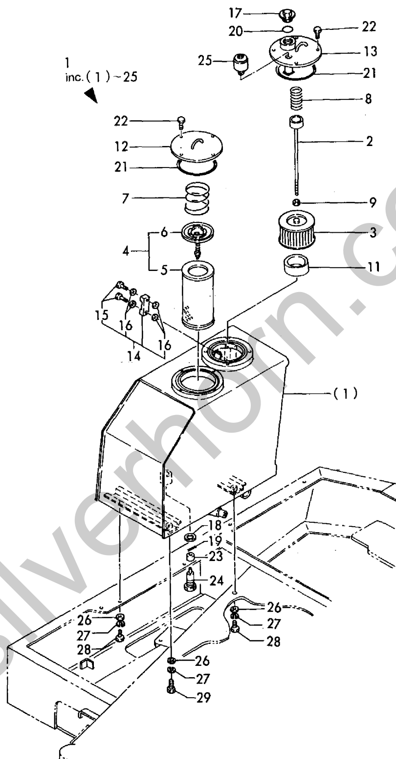
Fig. 59 サドウユタンク HYD. OIL TANK
