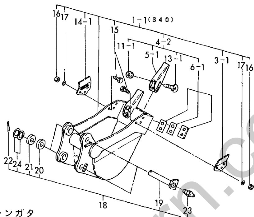
Fig. 72 バケット(300, 340)(アタッチメント) BUCKET(300, 340)(ATTACHMENT)
