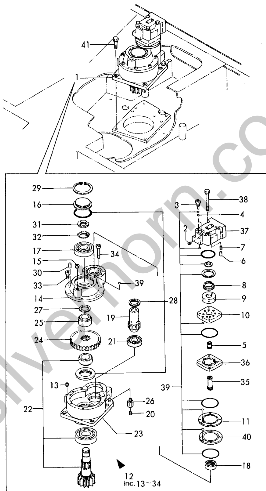
Fig. 48 センカイモータ TURNING MOTOR
