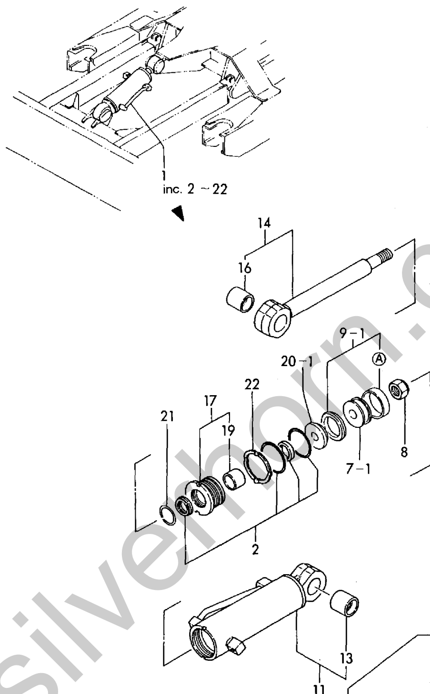
Fig. 46 ブレードシリンダ BLADE CYLINDER
