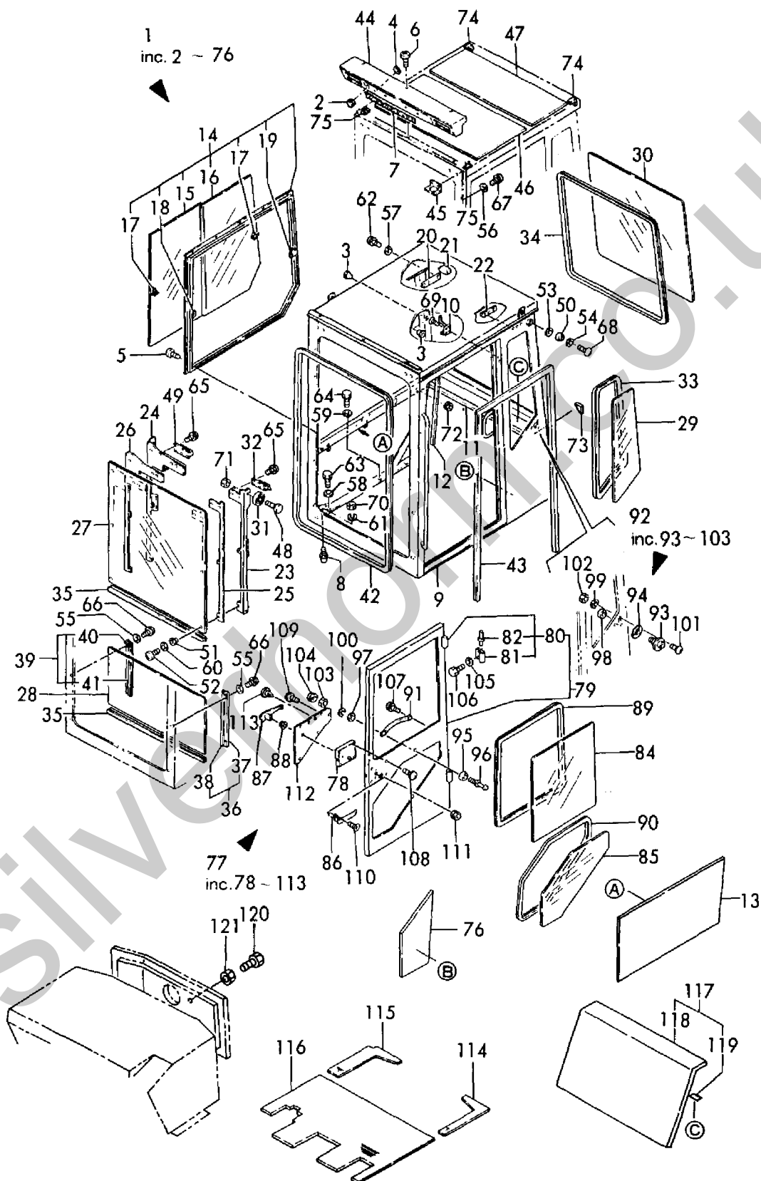
Fig. 37 キャビン CABIN
