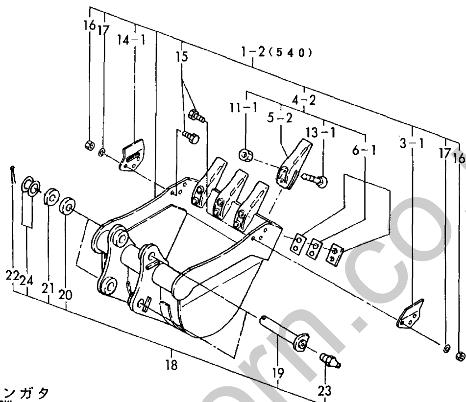
Fig. 74 バケット(500, 540)(アタッチメント) BUCKET(500, 540)(ATTACHMENT)
