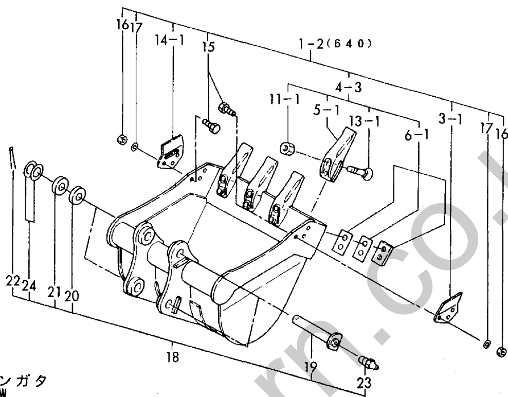
Fig. 75 バケット(600, 640)(アタッチメント) BUCKET(600, 640)(ATTACHMENT)
