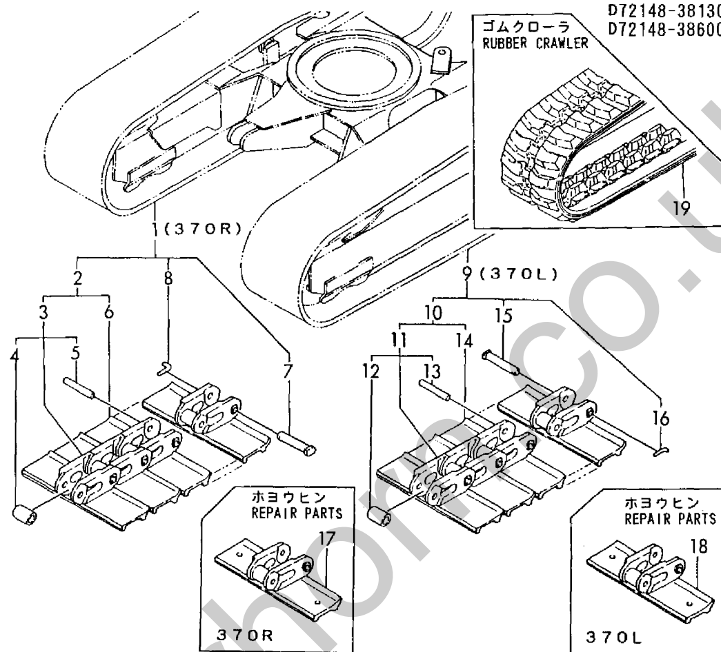
Fig. 19 クローラ CRAWLER
