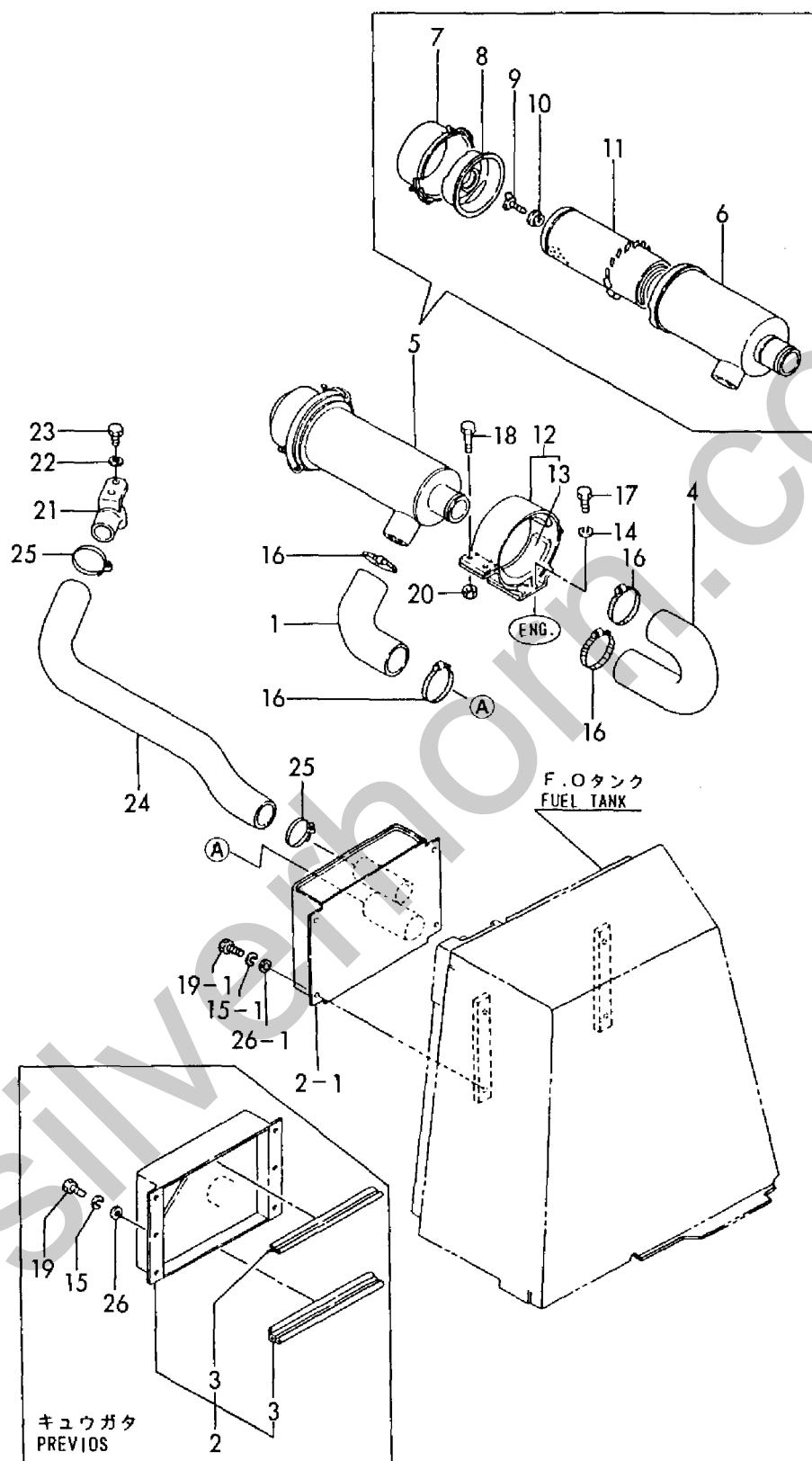
Fig. 7 エアクリーナ AIR CLEANER
