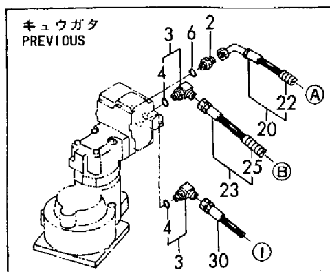
Fig. 61 ユアツハイカン(バルブ-モーター-ブーム) HYD. OIL PIPING (VALVE-MOTOR-BOOM)
